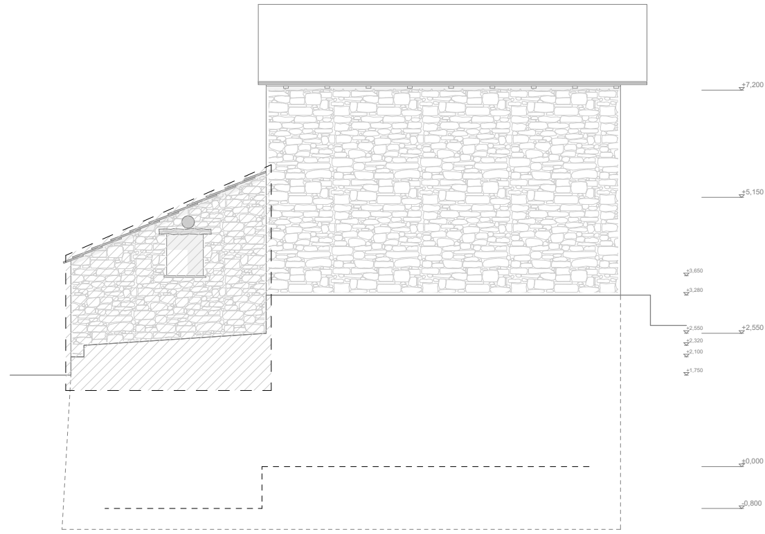
Prospetto Ovest
