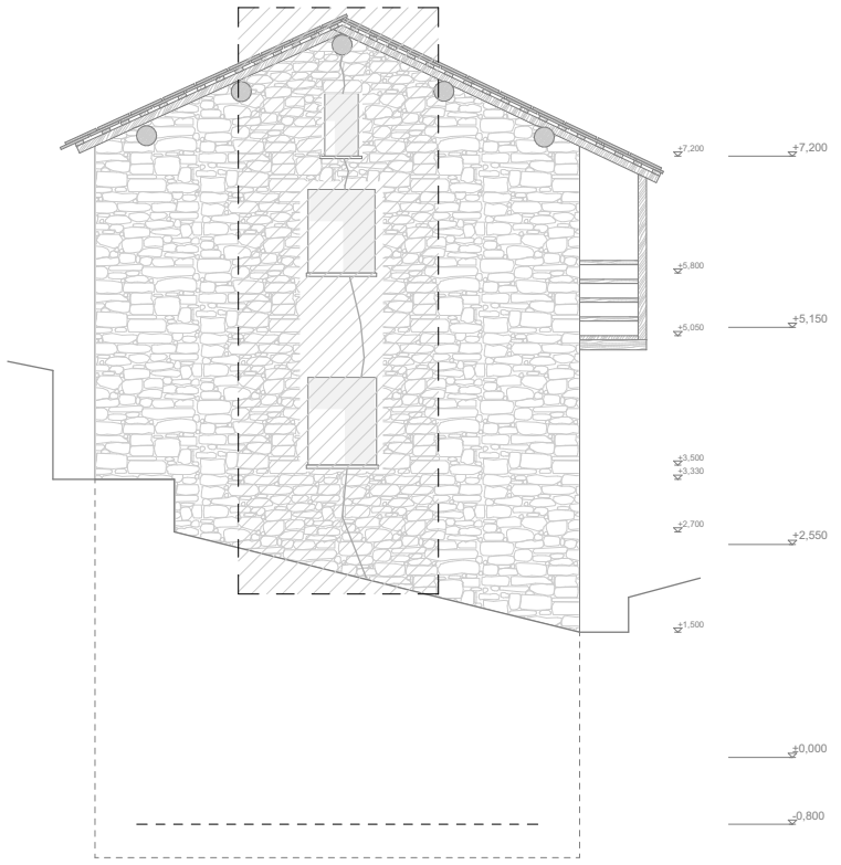
Prospetto Sud
