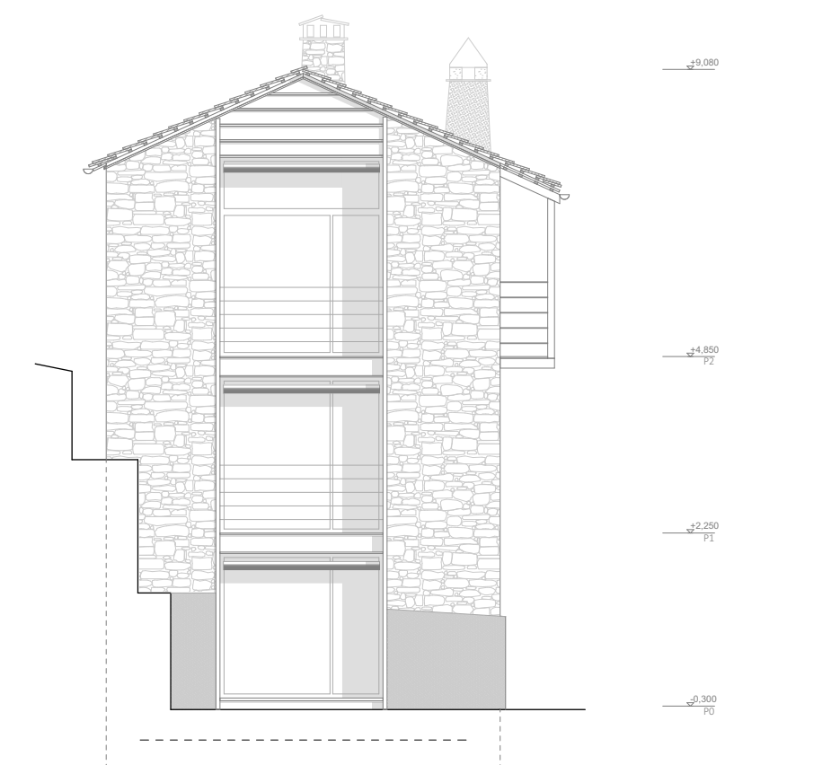
Prospetto Sud
