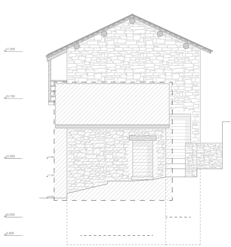
Prospetto Nord
