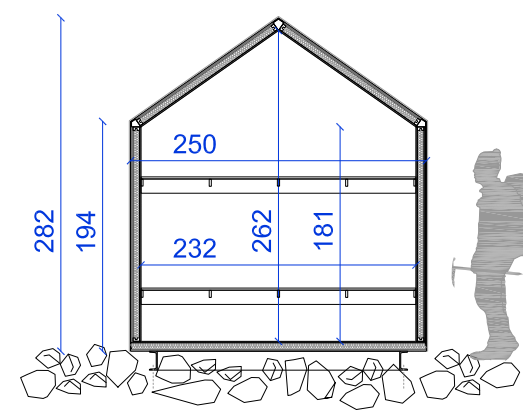
Sezione AA
