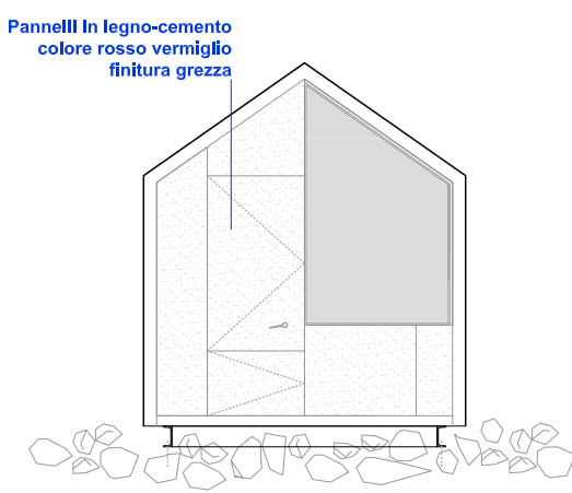
Prospetto / fronte
