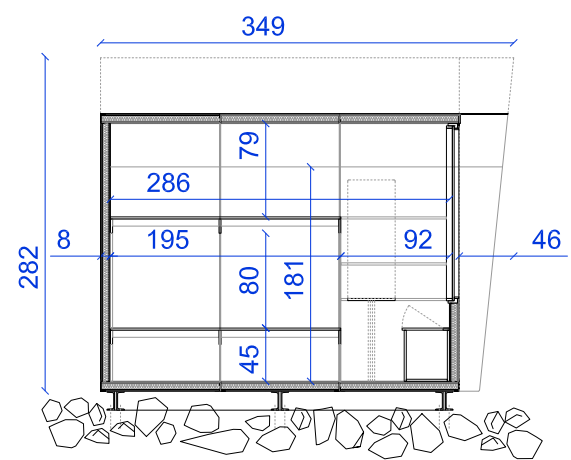
Sezione BB
